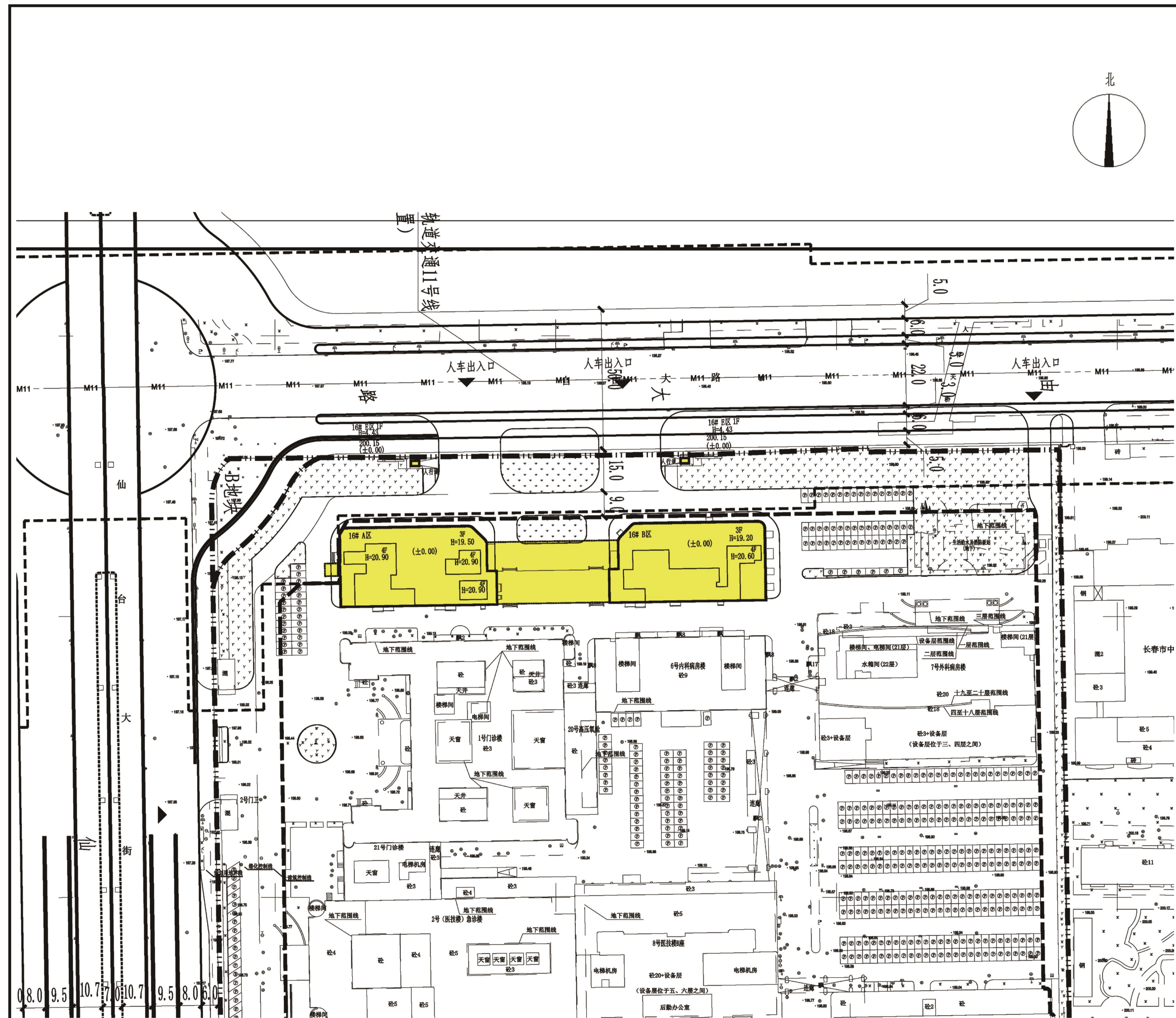
规划总平面图
